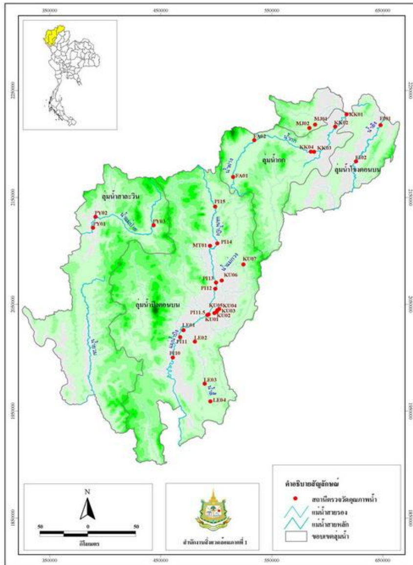
ภาพที่ 11 สถานีตรวจวัดคุณภาพน้ำในเขตจังหวัดเชียงราย
