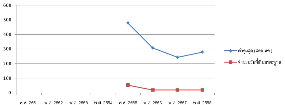
แผนภูมิที่ 33 แผนภูมิแสดงปริมาณฝุ่นละอองในบรรยากาศที่มีขนาดเล็กกว่า 10 ไมครอน (PM 10 ) และจำนวนวันที่เกินมาตรฐาน ของสถานีหน้าสำนักงานสาธารณสุขอำเภอแม่สาย
