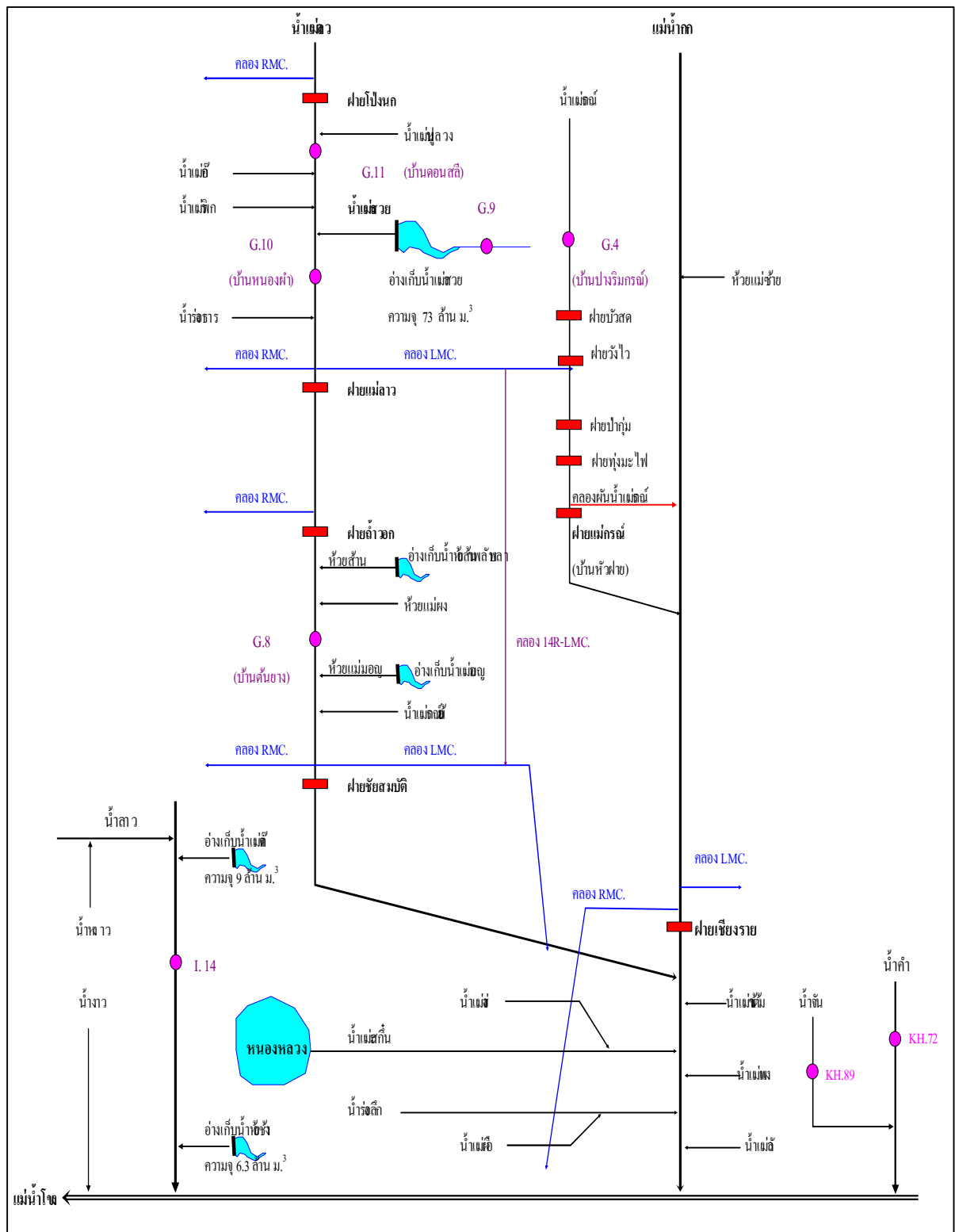
ภาพที่ 10 แหล่งน้ำที่สำคัญของจังหวัดเชียงราย
