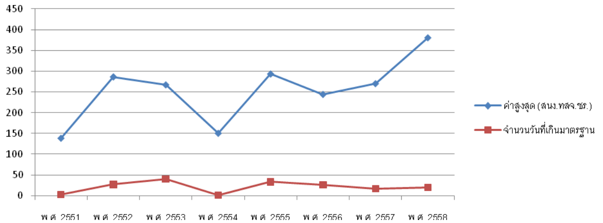
แผนภูมิที่ 32 แผนภูมิแสดงปริมาณฝุ่นละอองในบรรยากาศที่มีขนาดเล็กกว่า 10 ไมครอน (PM 10 ) และจำนวนวันที่เกินมาตรฐาน ของสถานีหน้าสำนักงานทรัพยากรธรรมชาติและสิ่งแวดล้อม จังหวัดเชียงราย
