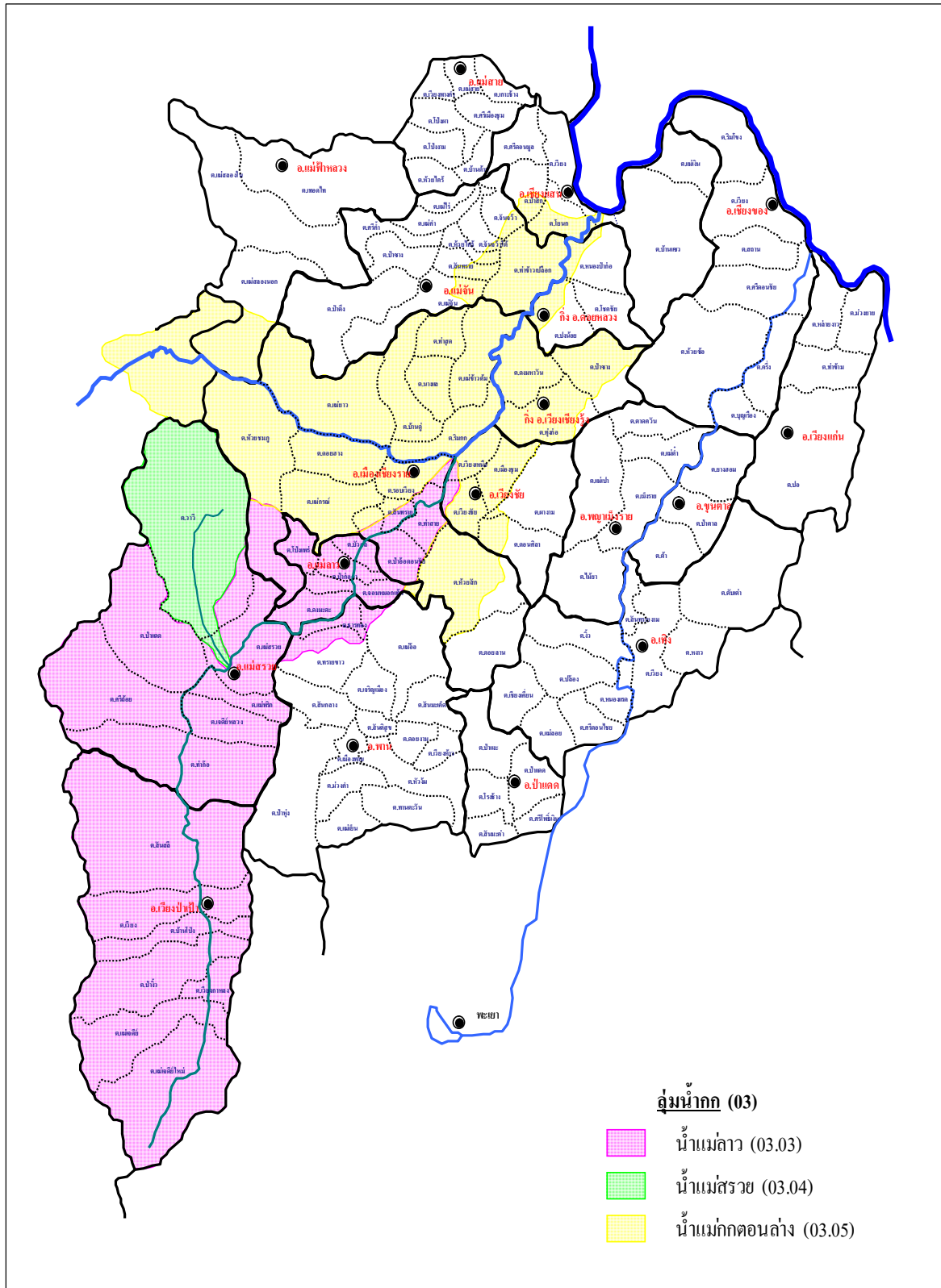
ภาพที่ 9 ลุ่มน้ำกก
