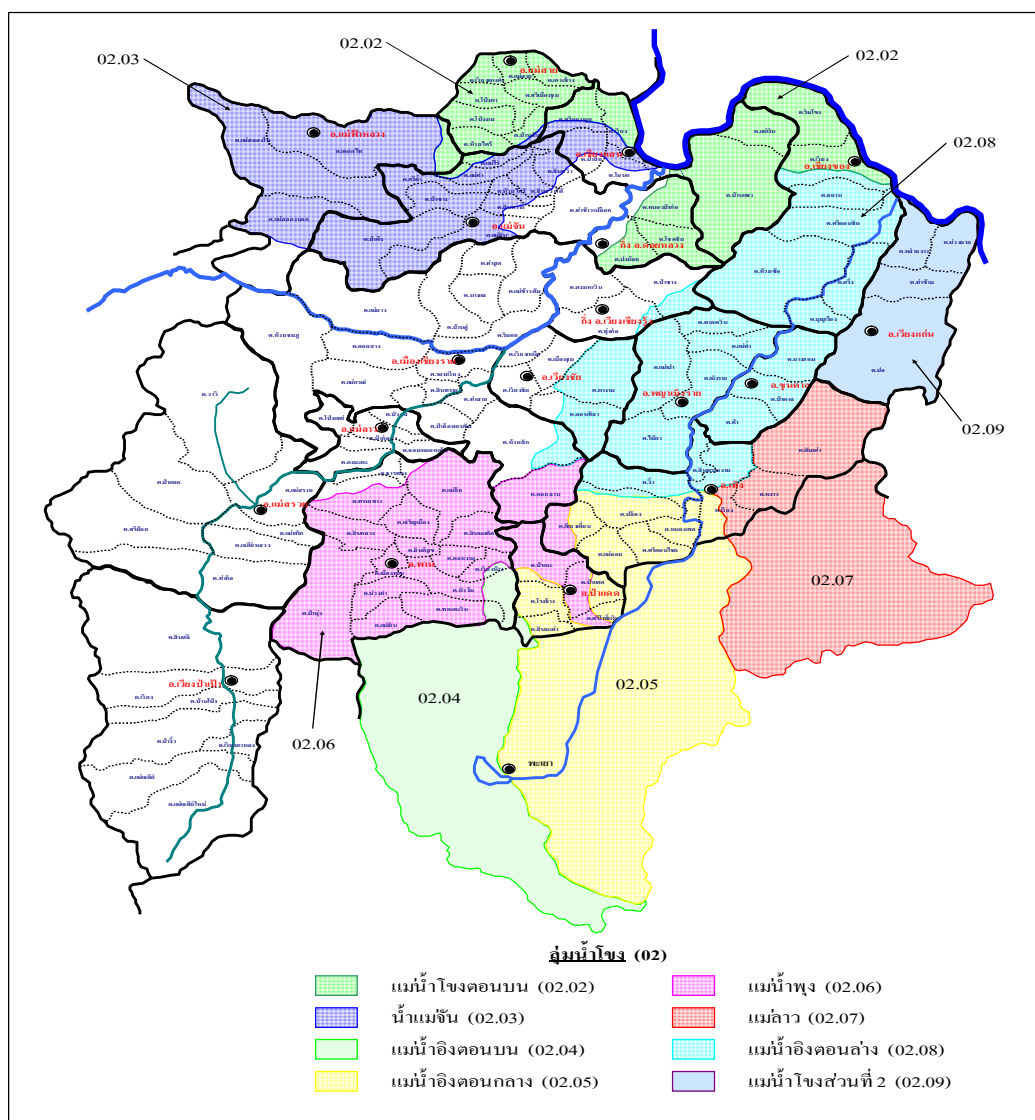
ภาพที่ 8 ลุ่มน้ำโขงเหนือ
