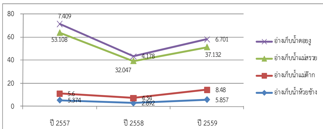
แผนภูมิที่ 28 ประมาณน้ำในอ่างเก็บน้ำขนาดกลาง ปี พ.ศ. 2557 – 2559 (ล้าน ลบ.ม.)
