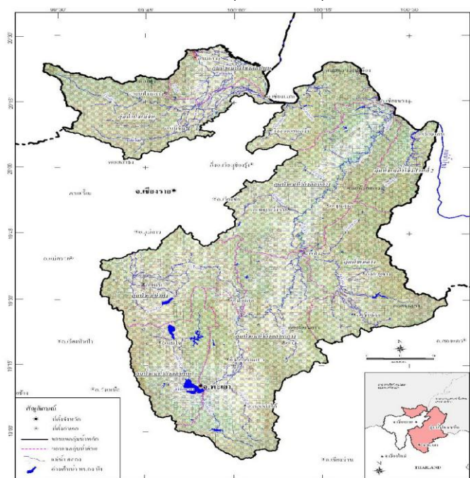
ภาพที่ 5 แสดงขอบเขตพื้นที่กลุ่มน้ำสาขากลุ่มน้ำโขง (ภาคเหนือ)
