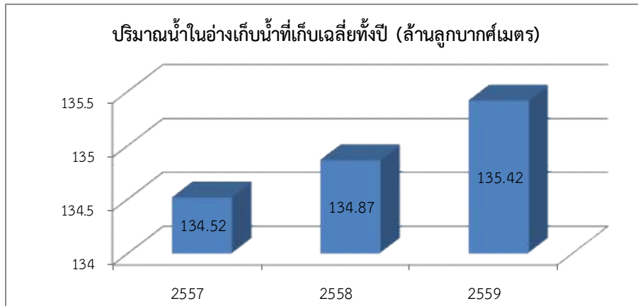
แผนภูมิที่ 30 ปริมาณน้ำในอ่างเก็บน้ำที่เก็บเฉลี่ยทั้งปี จำแนกตามรายอำเภอ พ.ศ. 2557 - 2559 (ล้านลูกบาศก์เมตร)
