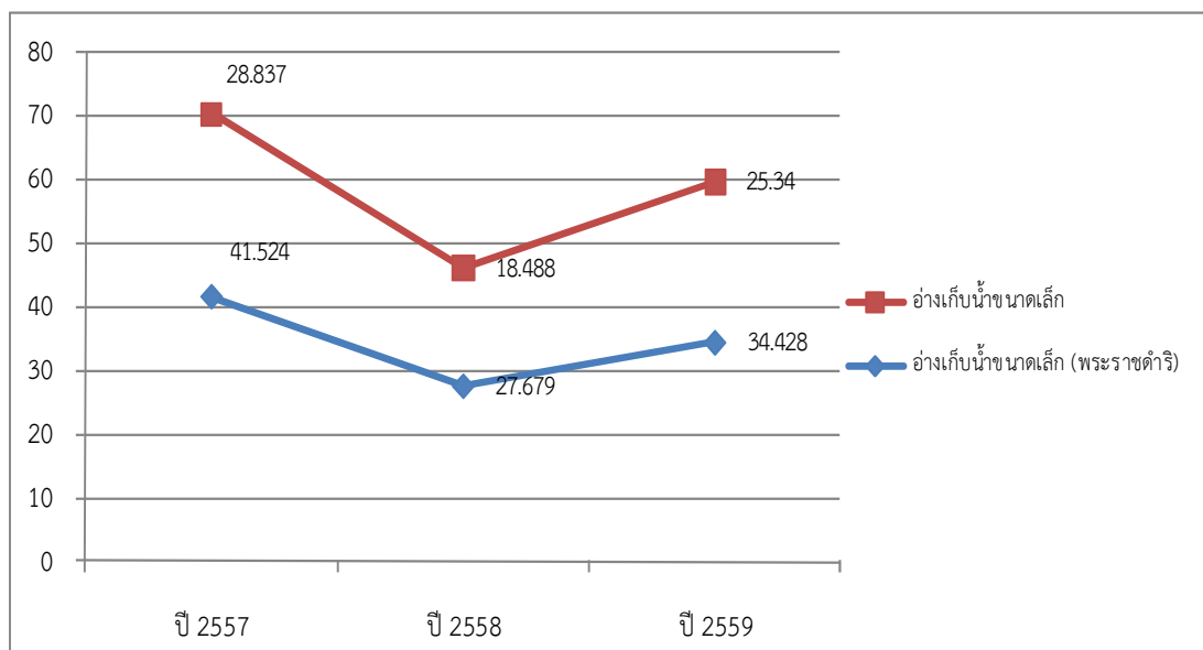
แผนภูมิที่ 29 ปริมาณน้ำในอ่างเก็บน้ำขนาดเล็ก ปี พ.ศ. 2557 – 2559 (ล้าน ลบ.ม.)
