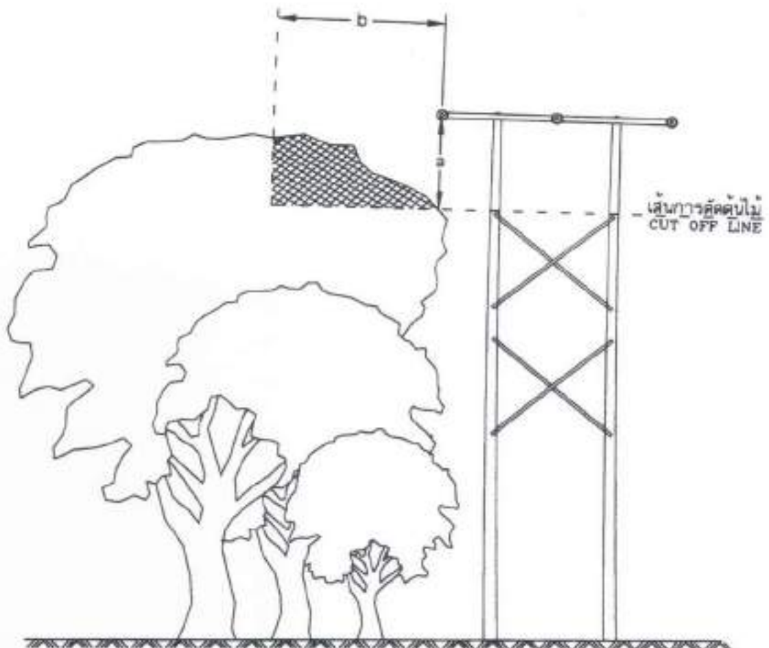
การตัดแต่งต้นไม้สำหรับสายเบ็ดเตล็ดแรงสูงที่มีระยะห่างระหว่างเสาตั้งแต่ 100 เมตร ขึ้นไป TREE TRIMMING FOR H.V. BARE CONDUCTOR WITH SPANS OF 100 m AND ABOVE.
