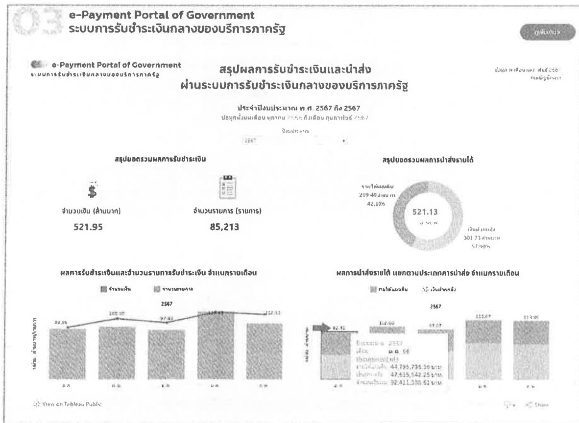
รูปที่ 14 หน้าจอเว็บไซต์หน้าภาพรวมของ e-Payment Portal of Government
