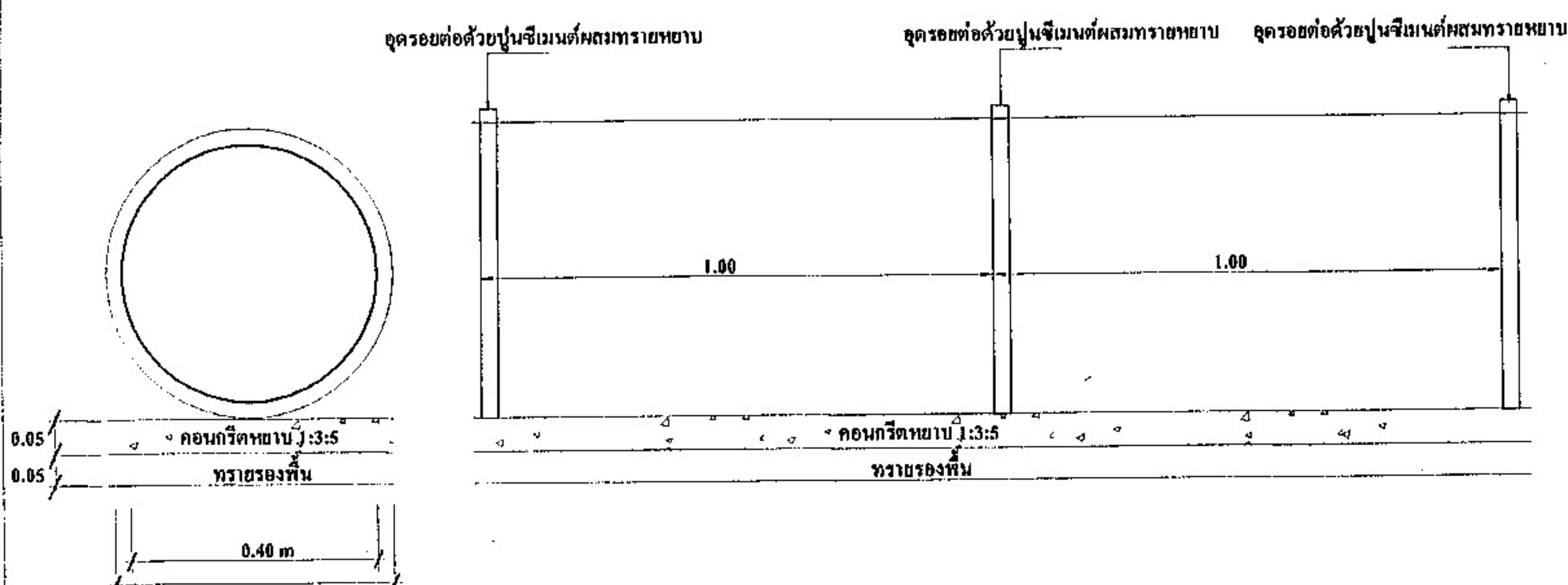
รูปตัด ท่อระบายน้ำ คสล.
