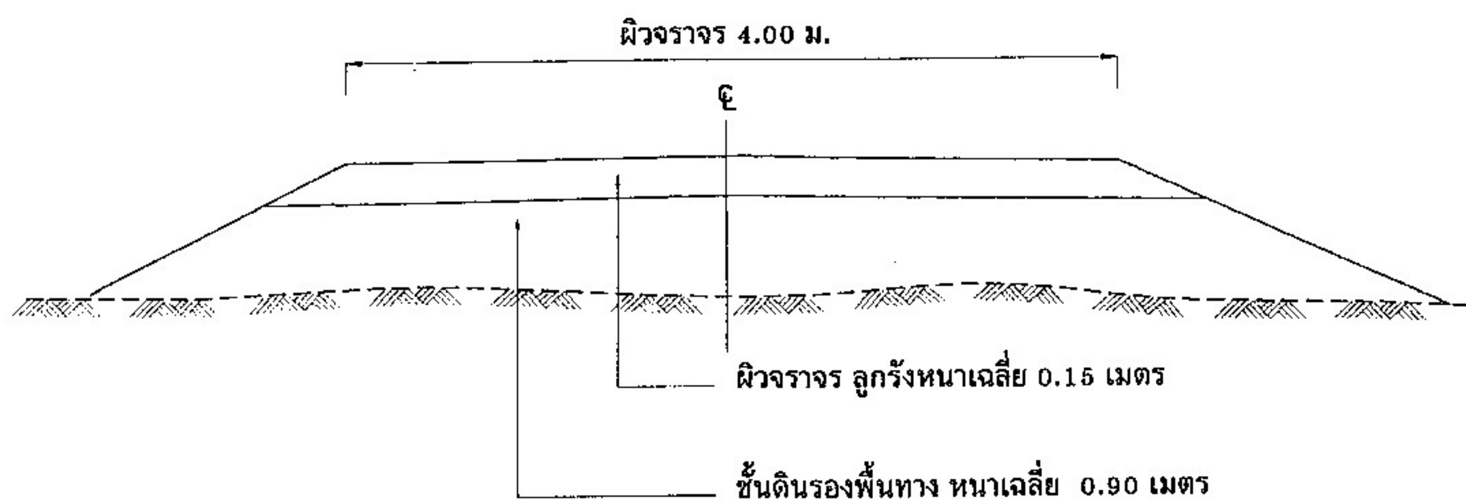
รูปตัดถนนดินลูกรัง
