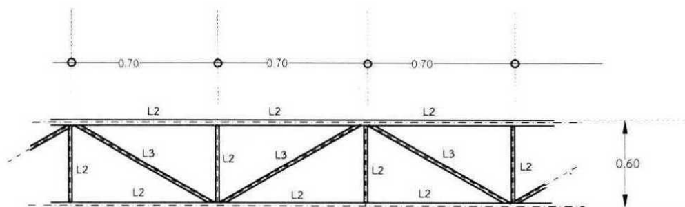
ขยายโครงถัก TRUSS 2 มาตรฐาน 1:25
