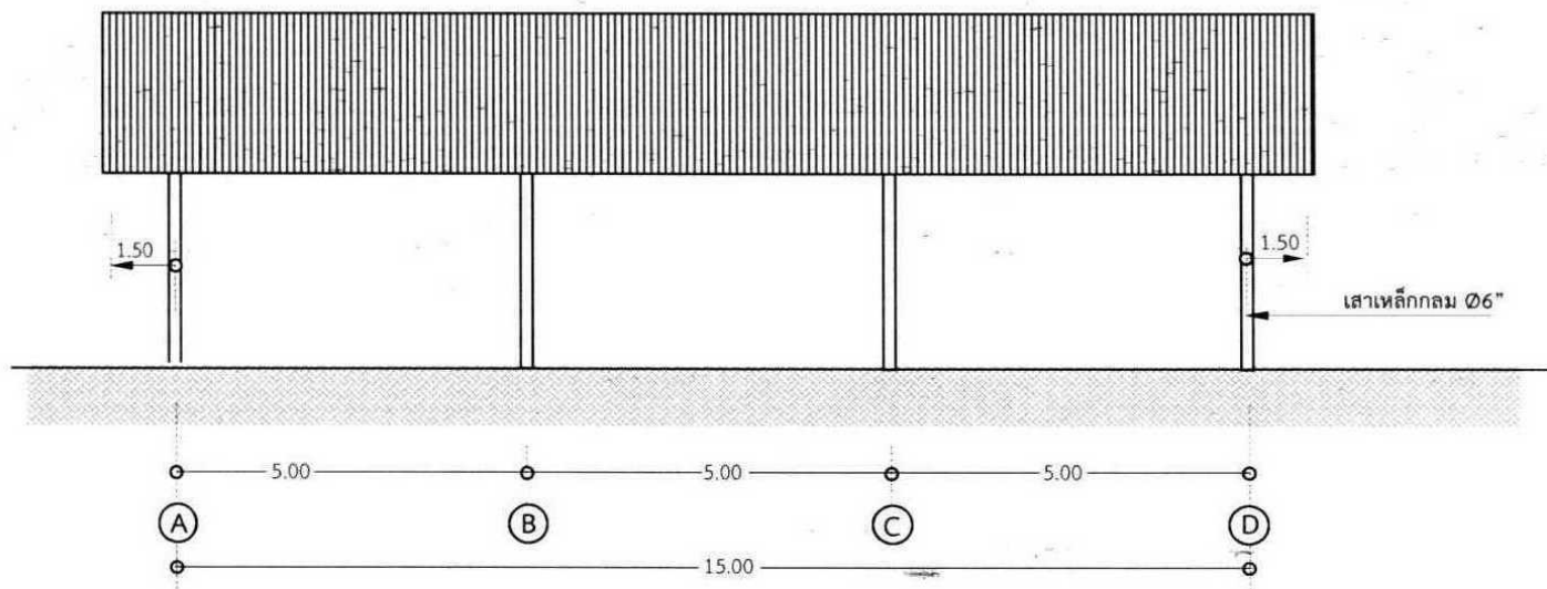
รูปด้าน C มาตราส่วน 1:100
