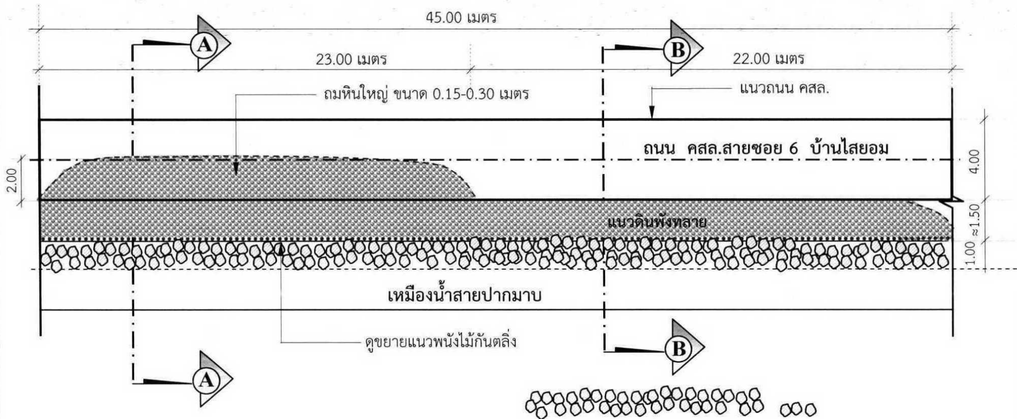
แปลนแสดงการซ่อมแซมไหล่ทางถนน คสล.ชำรุด มาตราส่วน 1:200
