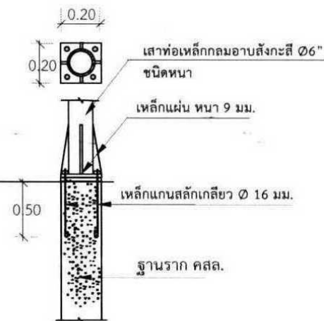
ขยาย A (จำนวน 8 ฐาน) มาตราส่วน 1:20
