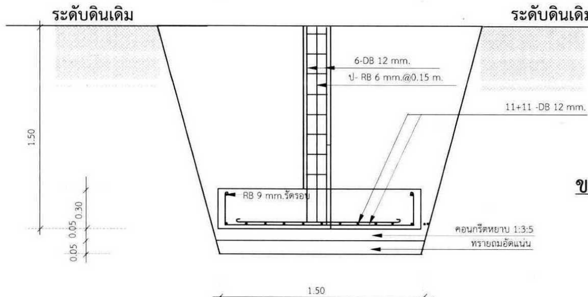
ขยายฐานราก F1,C1 มาตราส่วน 1:20
