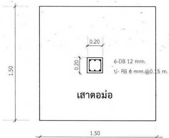
F1,C1 มาตราส่วน 1:20
