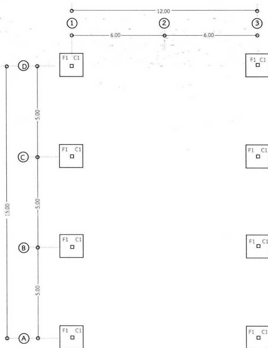
แปลนฐานราก ตอม่อ มาตราส่วน 1:100
