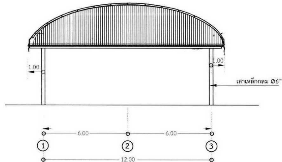
รูปด้าน B มาตราส่วน 1:100
