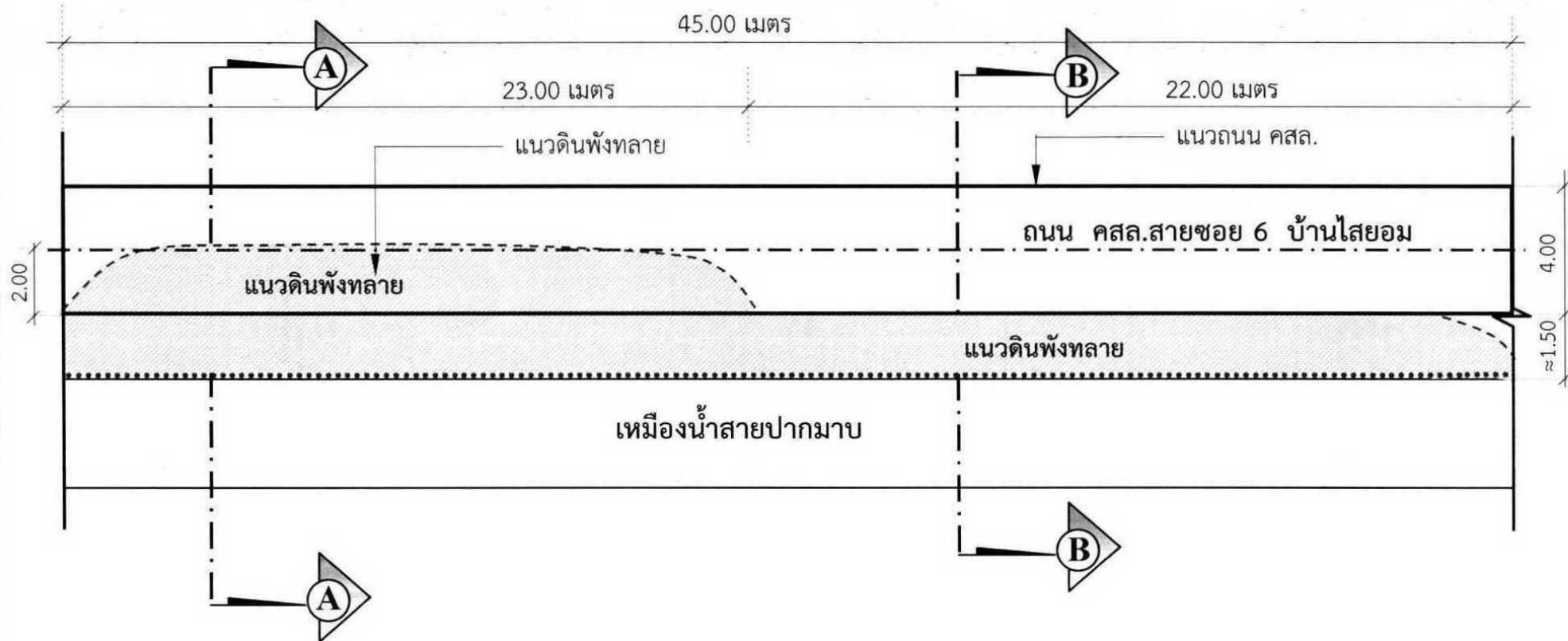
แปลนซ่อมแซมไหล่ทางถนน คสล.ชำรุด มาตราส่วน 1:200
