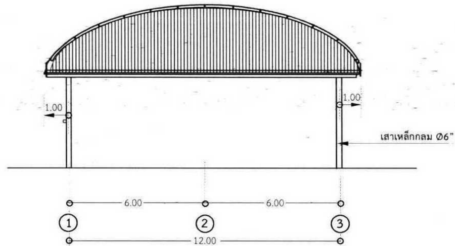
รูปด้าน A มาตราส่วน 1:100
