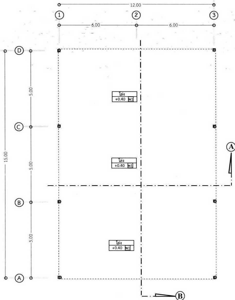
แปลนพื้น มาตราส่วน 1:100
