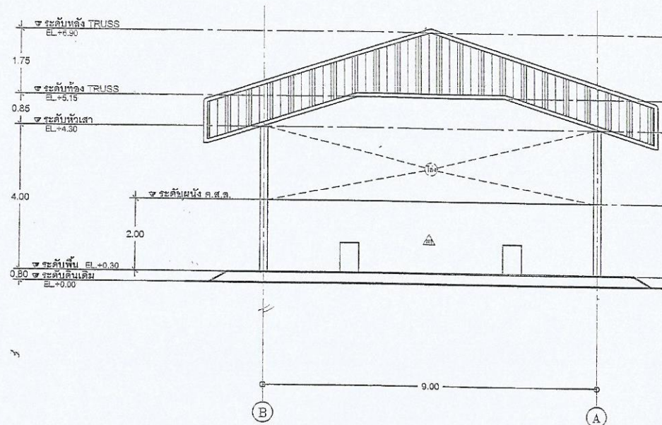
รูปด้านสาม มาตราส่วน 1/100
