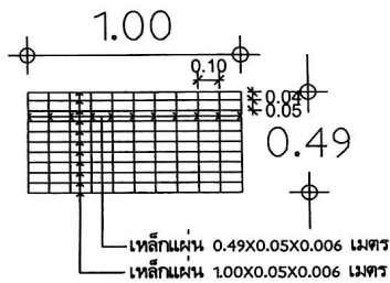
ขยายฝ่าตะแกรงเหล็ก NOT TO SCALE
