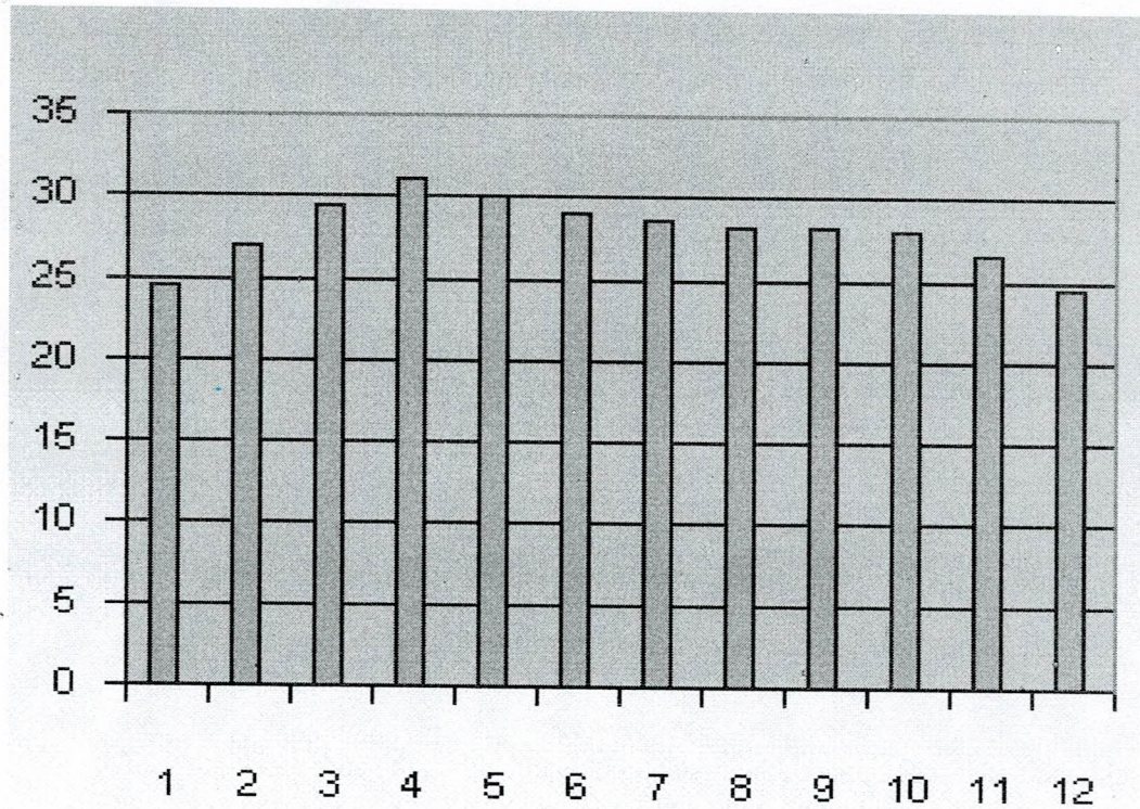
อุณหภูมิเฉลี่ยแต่ละเดือน ( องศาเซลเซียส )
