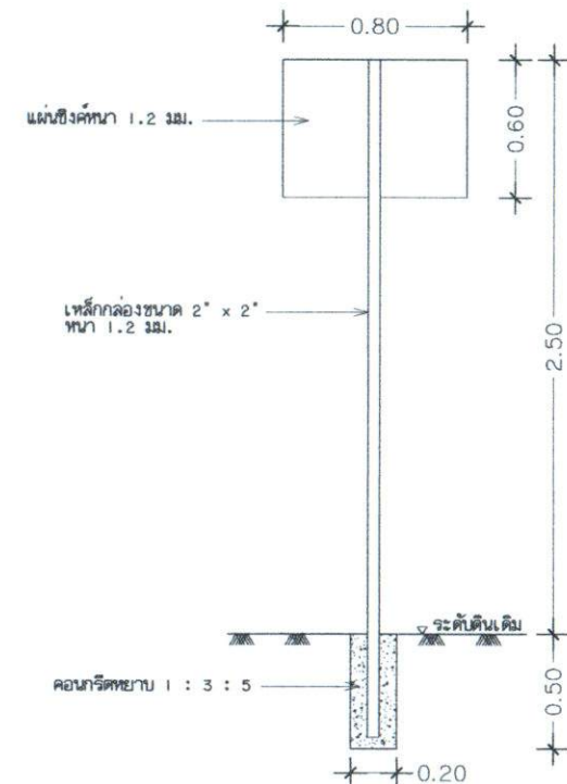
รูปตัดด้านหลังป้ายโครงการ (เหล็ก) มาตรฐาน 1:25
