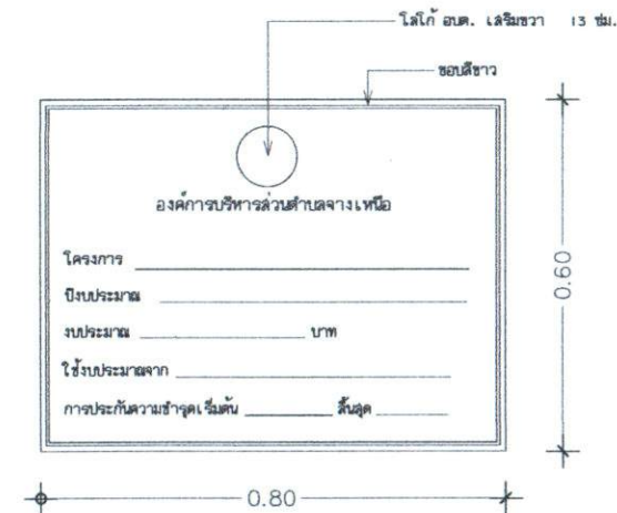
ภาพถ่ายข้อความในป้ายโครงการ (เหล็ก) มาตรฐาน 1:25
