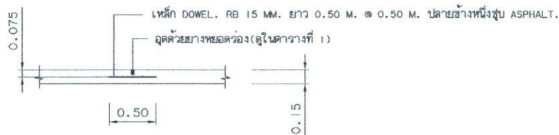
CONTRACTION JOINT มาตราส่วน 1 : 75
