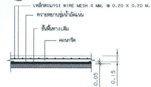
รายละเอียดถนนคอนกรีตเสริมเหล็ก มาตราส่วน 1 : 75
