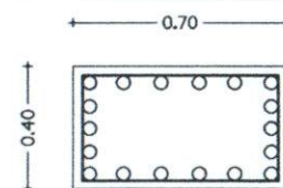
แบบขยาย C1
