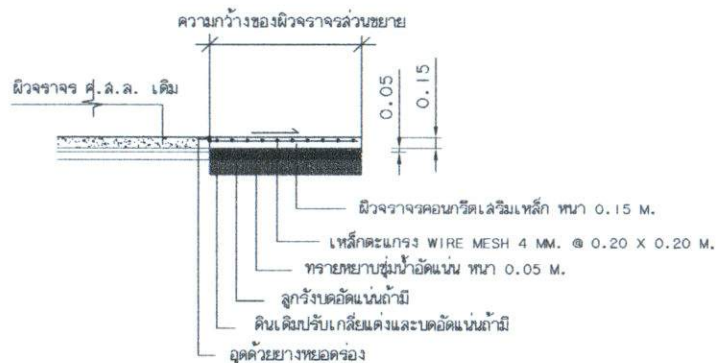
รูปตัดแฉ่งโครงสร้างถนนคอนกรีตเสริมเหล็ก กรณีขยายผิวจราจร ค.ล.ล.)
