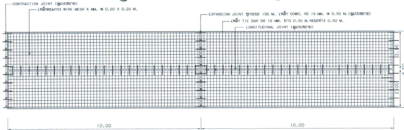
แผนการวางเหล็กตะแกรง
