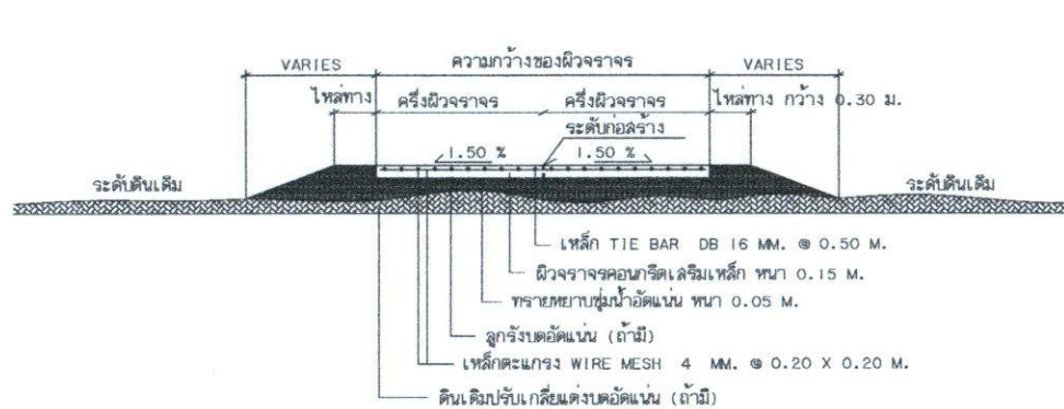
รูปตัดแสดงโครงสร้างถนนคอนกรีตเสริมเหล็ก
