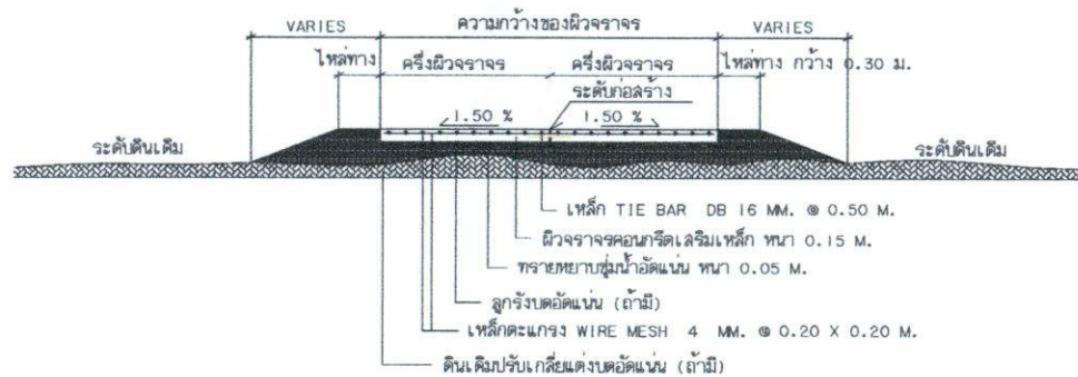
รูปตัดแฉ่งโครงสร้างถนนคอนกรีตเสริมเหล็ก
