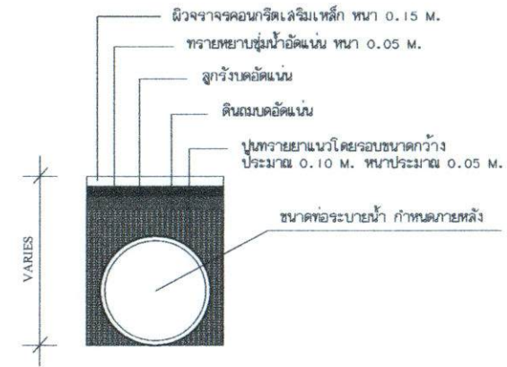
รูปตัดแสดงการวางท่อระบายน้ำ (กรณีการวางท่อลอดถนน)
