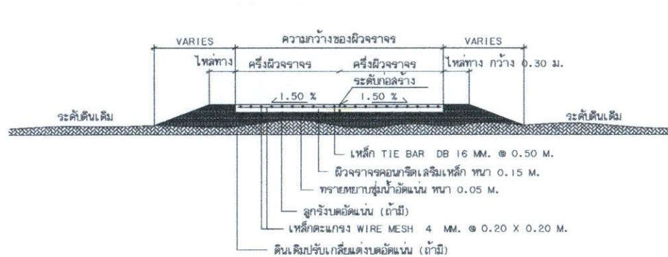
รูปตัดแฉ่งโครงสร้างถนนคอนกรีตเสริมเหล็ก
