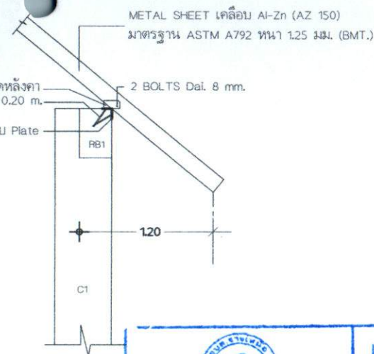
แบบขยายรอยต่อ 1
