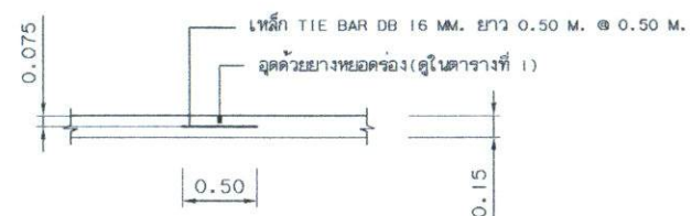
LONGITUDINAL JOINT มาตราส่วน 1 : 75
