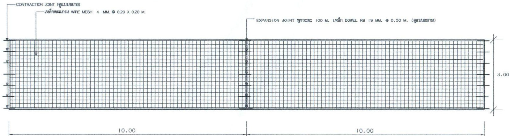
แปลนการวางเหล็กตะแกรง มาตราส่วน 1 : 75
