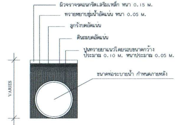
รูปตัดแสดงการวางท่อระบายน้ำ (กรณีการวางท่อลอดถนน)
