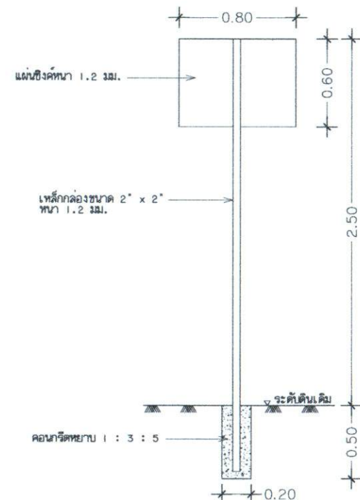
รูปตัดด้านหลังป้ายโครงการ (เหล็ก) มาตรฐาน 1:25
