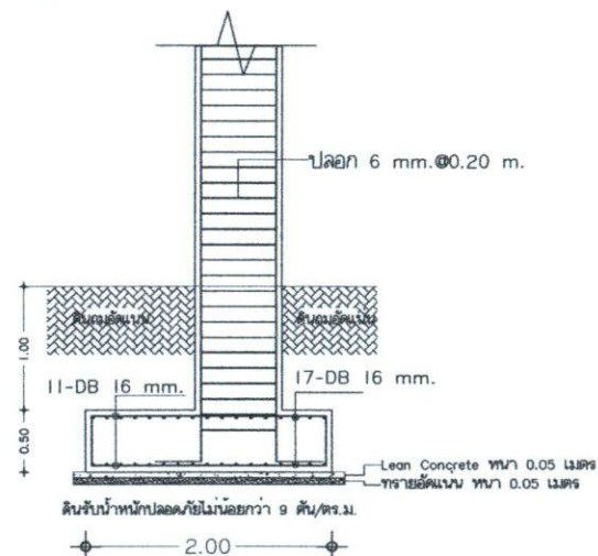
แบบฐานราก F1
