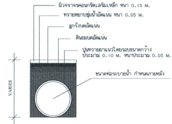
รูปตัดแฉ่งการวางท่อระบายน้ำ (กรณีการวางท่อลอดถนน)
