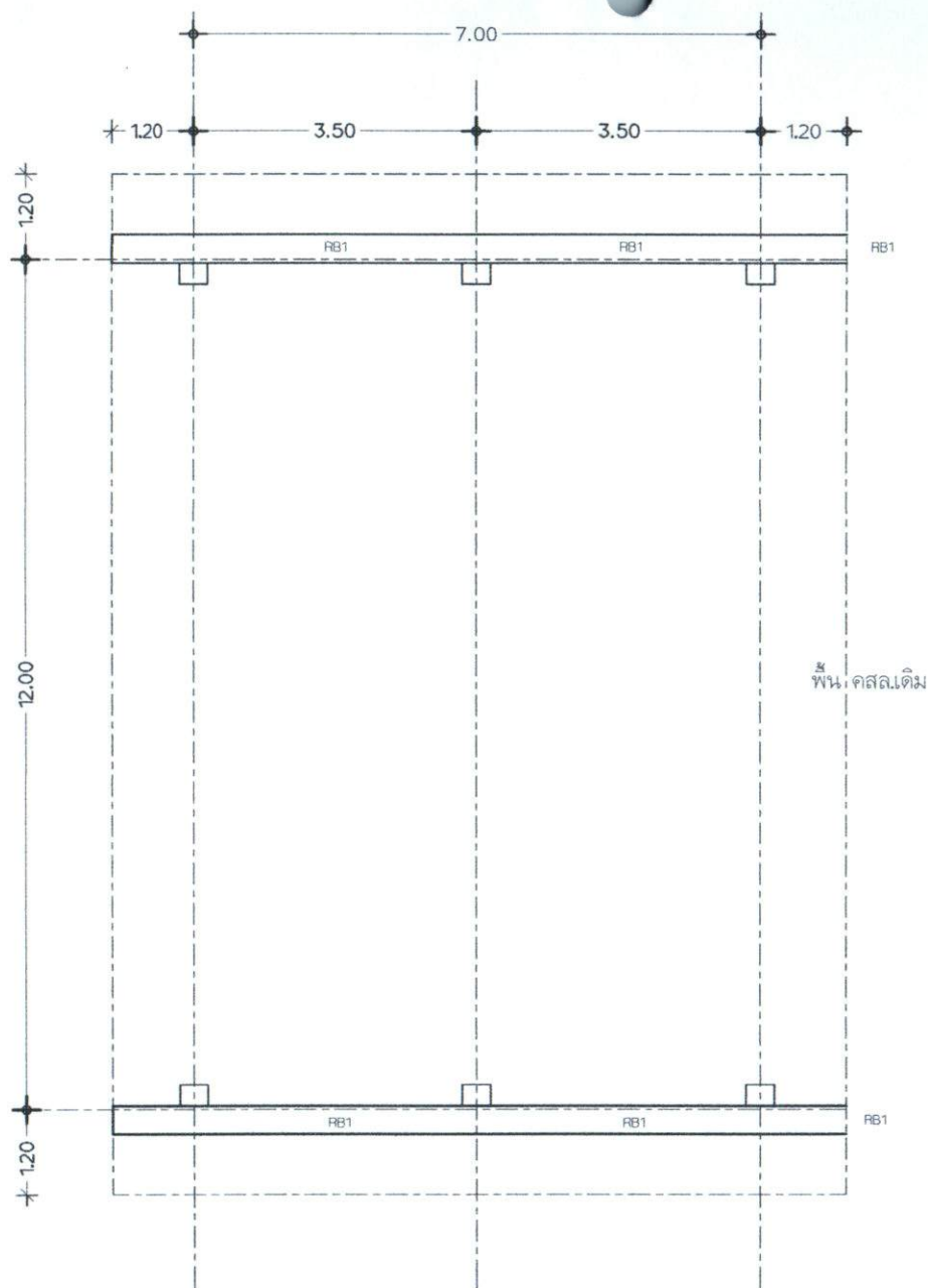
แปลนคานหลังคา
