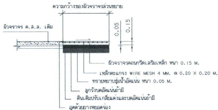
รูปตัดแสดงโครงสร้างถนนคอนกรีตเสริมเหล็ก กรณีขยายผิวจราจร ค.ล.ล.)
