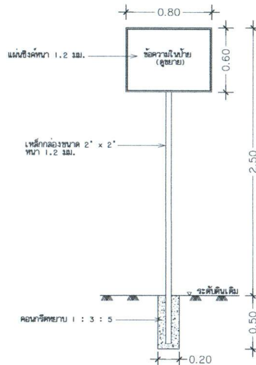
รูปตัดด้านหน้าป้ายโครงการ (เหล็ก) มาตรฐาน 1:25
