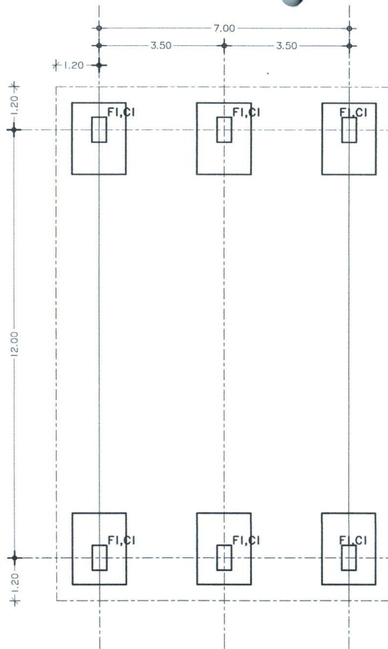
แปลนพื้น ฐานราก
