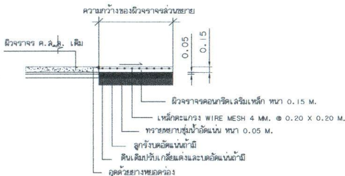
รูปตัดแฉ่งโครงสร้างถนนคอนกรีตเสริมเหล็ก กรณีขยายผิวจราจร ค.ล.ล.)
