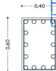
แบบขยาย RB1
