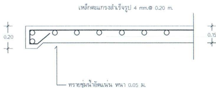
แบบขยายพน GS
