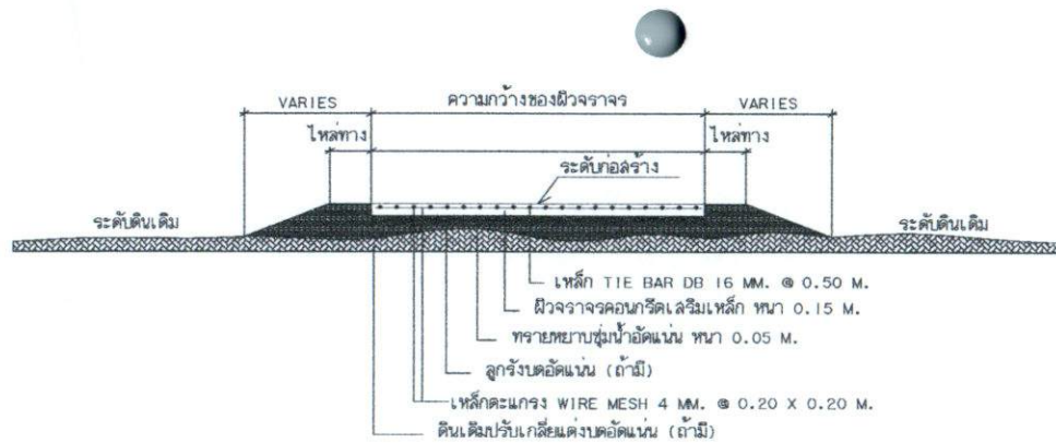
รูปตัดแฉ่งโครงสร้างถนนคอนกรีตเสริมเหล็ก
