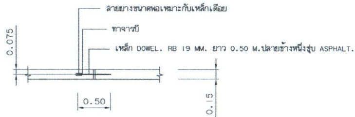
EXPANSION JOINT มาตราส่วน 1 : 75
