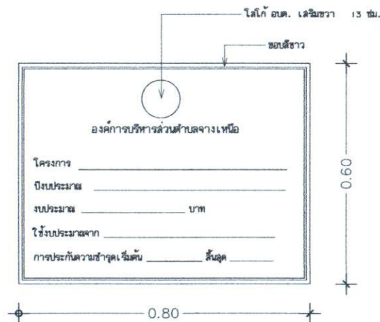
ภาพถ่ายข้อความในป้ายโครงการ (เหล็ก) มาตรฐาน 1:25
