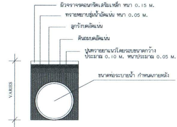
รูปตัดแฉ่งการวางท่อระบายน้ำ (กรณีการวางท่อลอดถนน)
