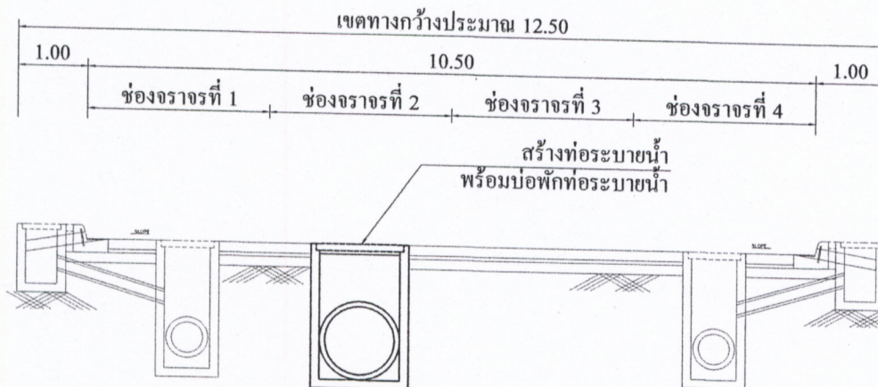
รูปตัดถนน-1 SCALE 1 : 100
